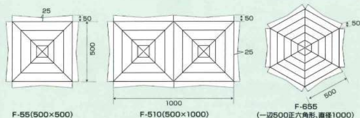
● F-655 (一辺500正六角形、直径1000)
